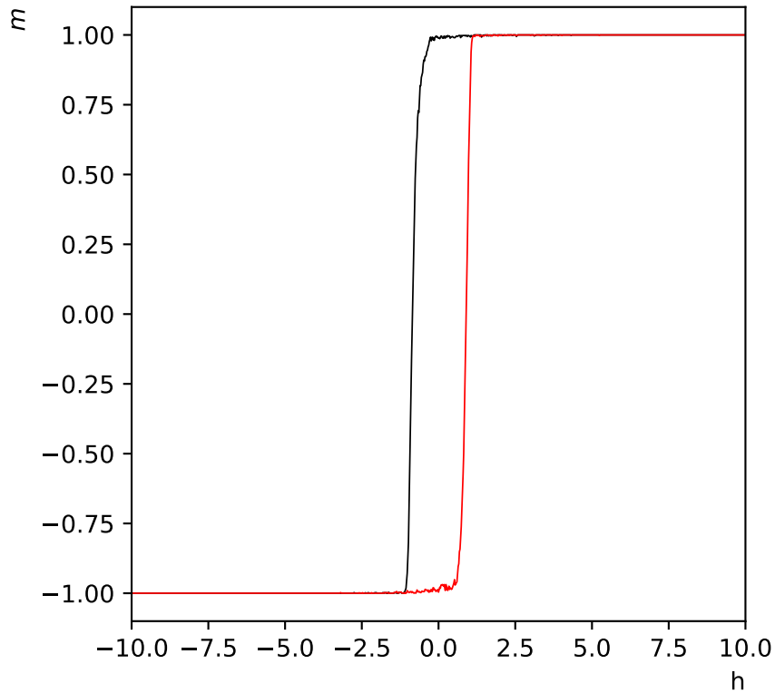
Hystérésis de l'aimantation réseau de taille L=32 - h=10 à T=1.5
